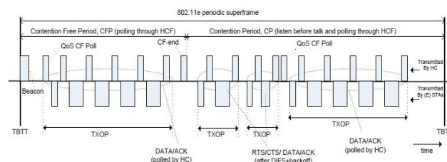
Fig. 3. IEEE 802.11e periodic superframe
